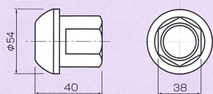
球面ナット
